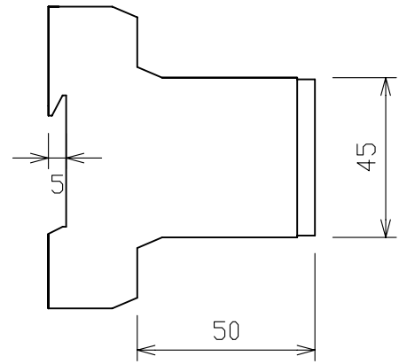
左側面図
